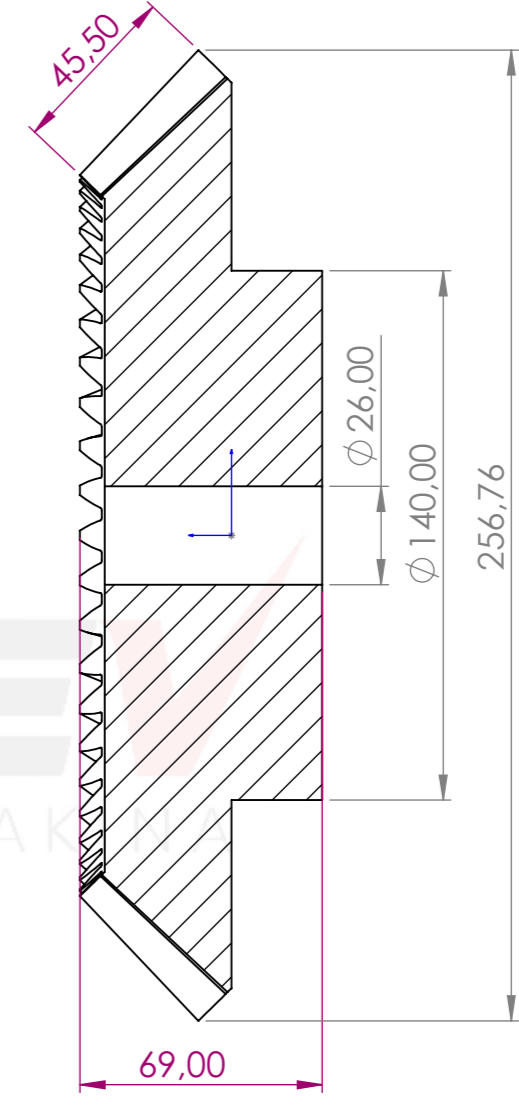
KESIT A-A
