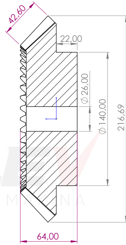
KESİT A-A
