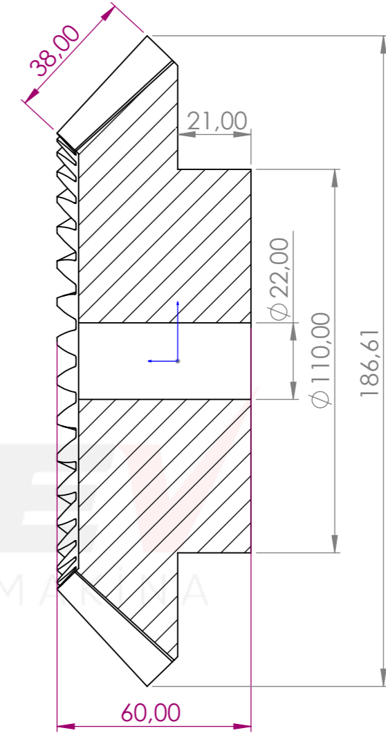
KESIT B-B ÖLÇEK 1 : 1.5
