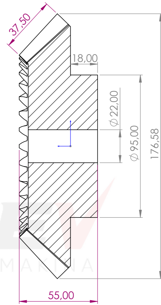
KESİT A-A ÖLÇEK 1 : 1.5
