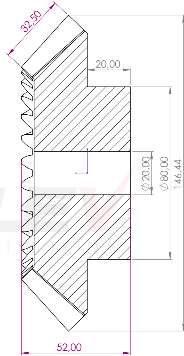
KESİT A-A ÖLÇEK 1 : 1
