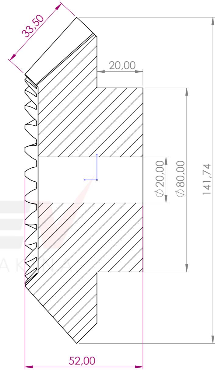
KESİT A-A ÖLÇEK 1 : 1
