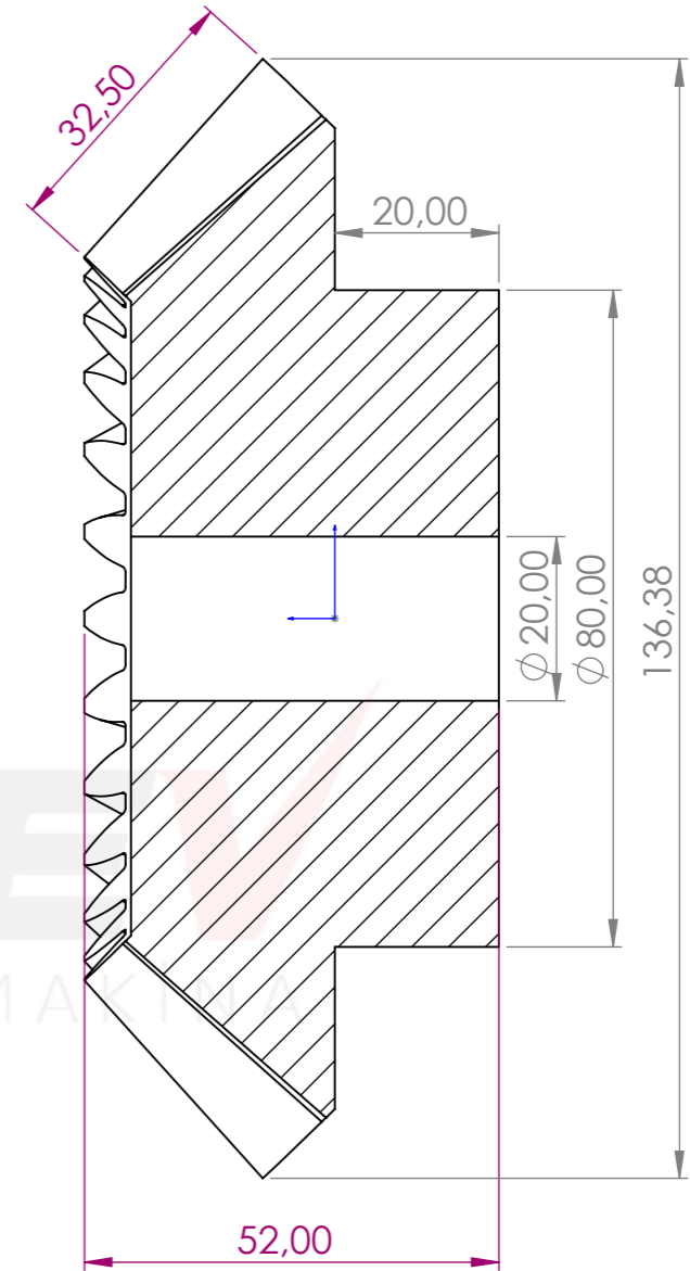
KESİT A-A ÖLÇEK 1 : 1
