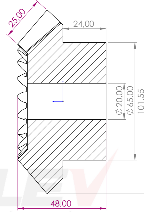
KESİT A-A
