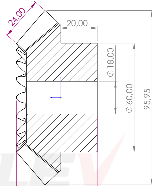
KESİT A-A
