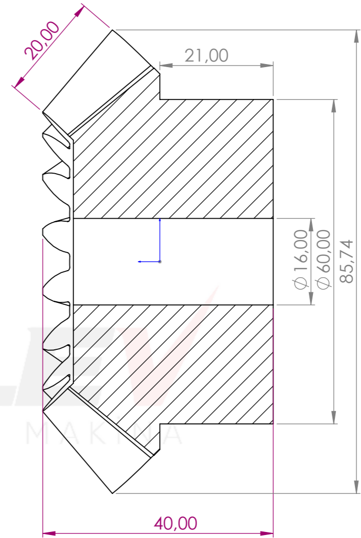
KESİT A-A ÖLÇEK 2 : 1.4
