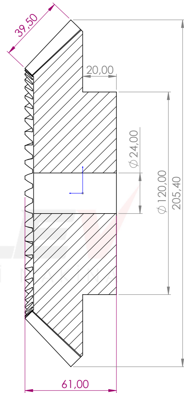
KESİT A-A ÖLÇEK 1 : 1.4
