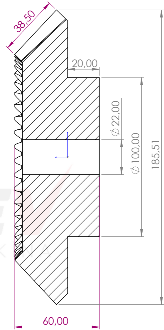
KESİT A-A ÖLÇEK 1 : 1.4
