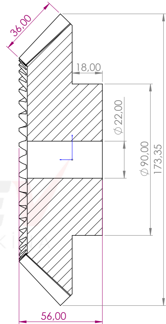
KESİT A-A ÖLÇEK 1 : 1.3
