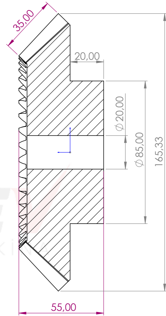
KESİT A-A ÖLÇEK 1 : 1.3
