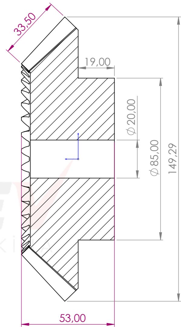
KESİT A-A ÖLÇEK 1 : 1.2
