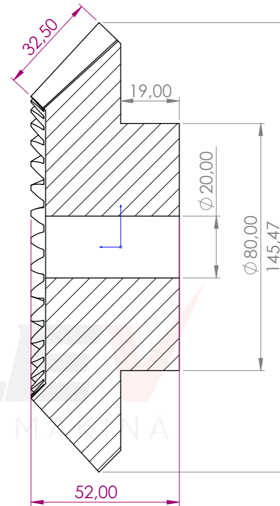
KESİT A-A ÖLÇEK 1 : 1.2
