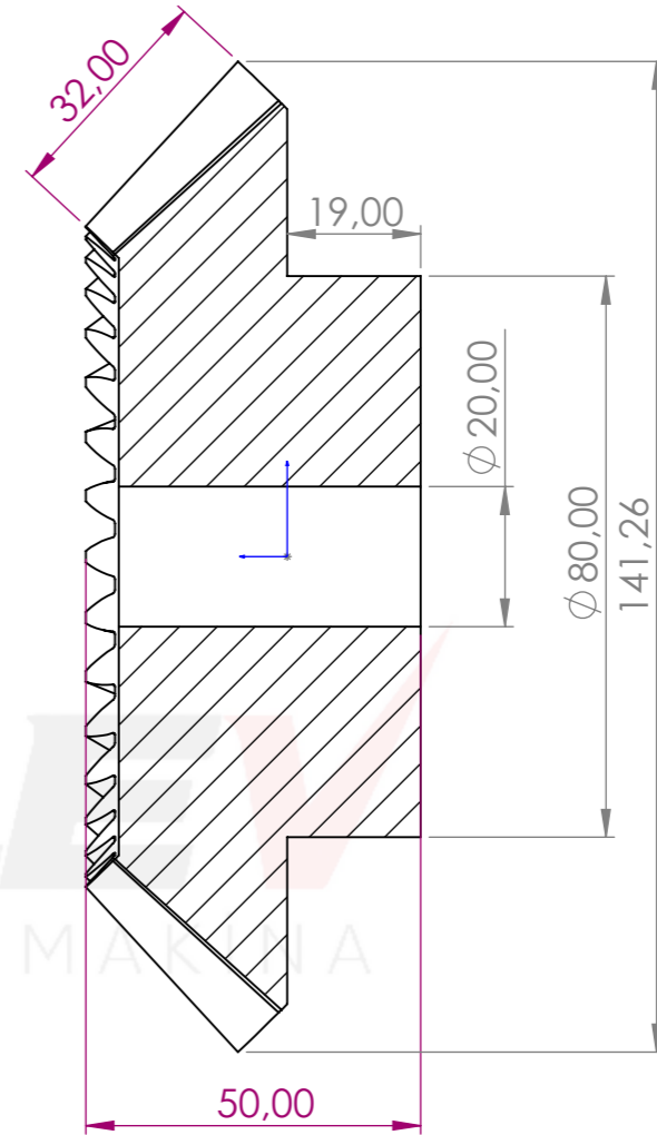
KESİT A-A ÖLÇEK 1 : 1.2
