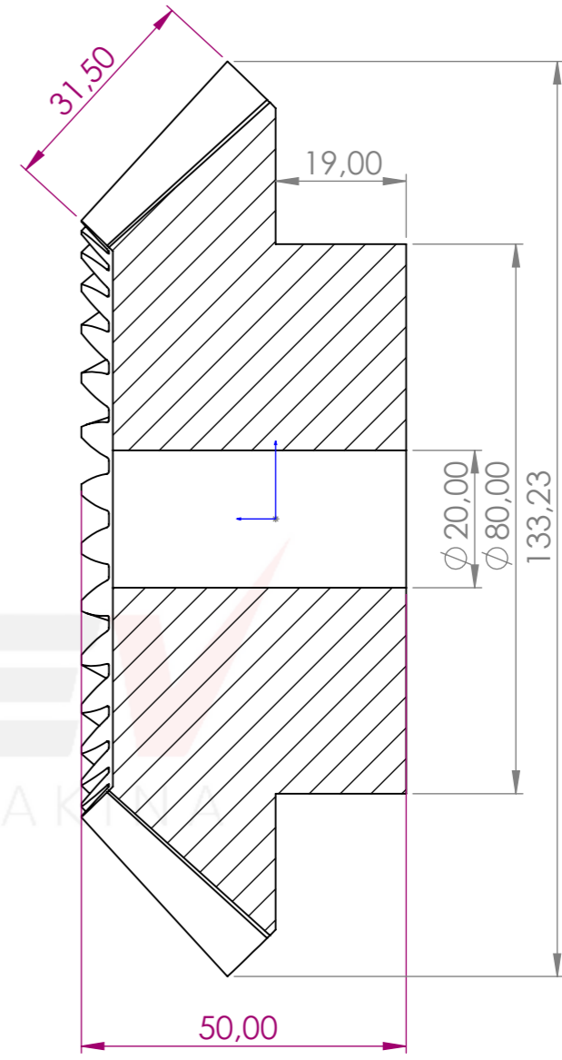
KESİT A-A ÖLÇEK 1 : 1
