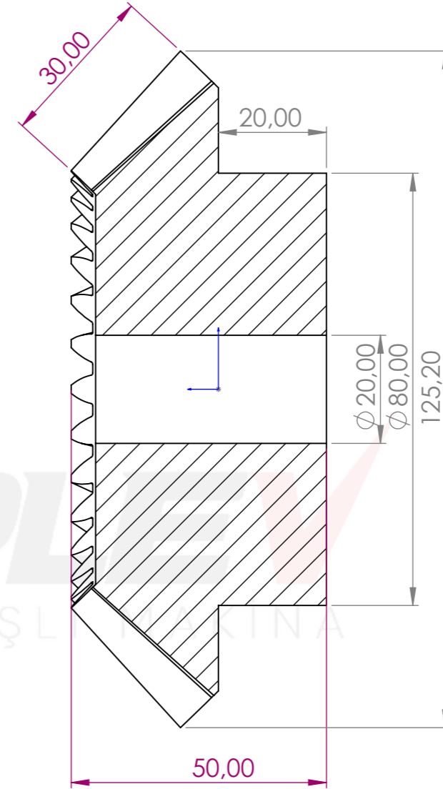
KESİT A-A ÖLÇEK 1 : 1
