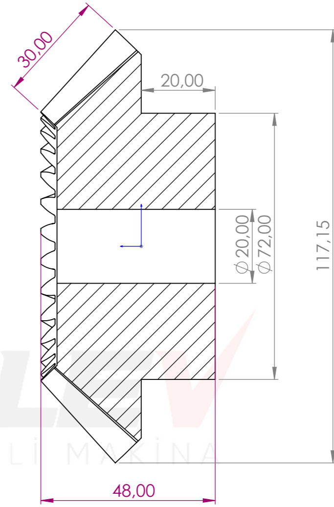
KESİT A-A ÖLÇEK 1 : 1
