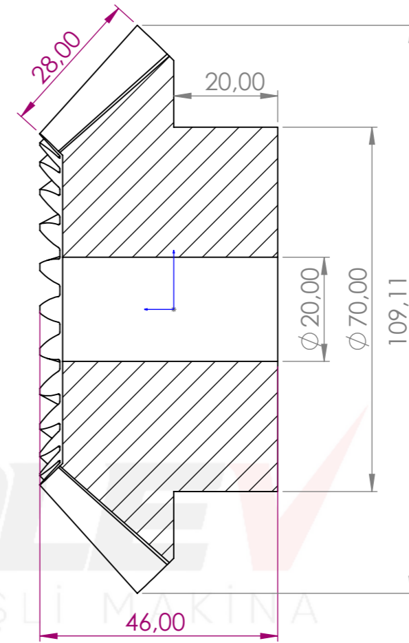
KESIT A-A
