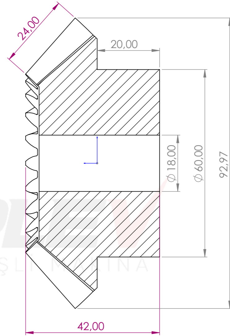
KESİT A-A ÖLÇEK 2 : 1.5
