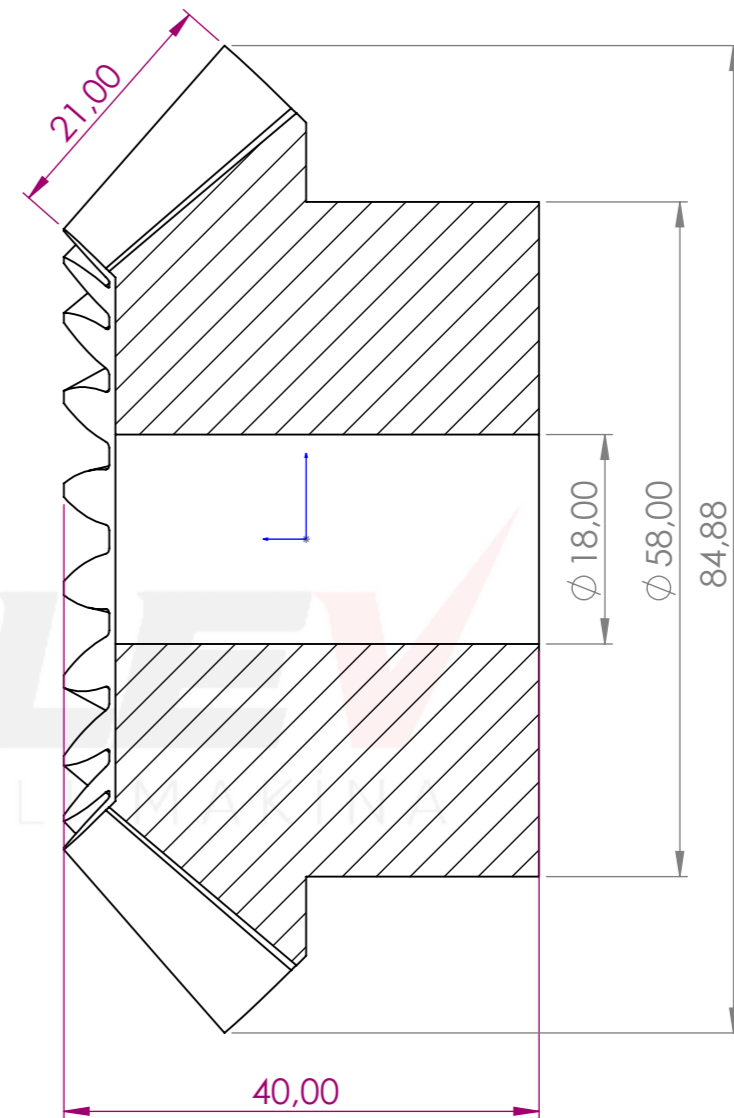
KESİT A-A ÖLÇEK 2 : 1.3
