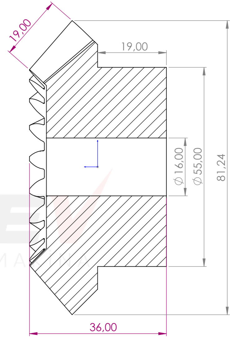
KESİT A-A ÖLÇEK 2 : 1.3
