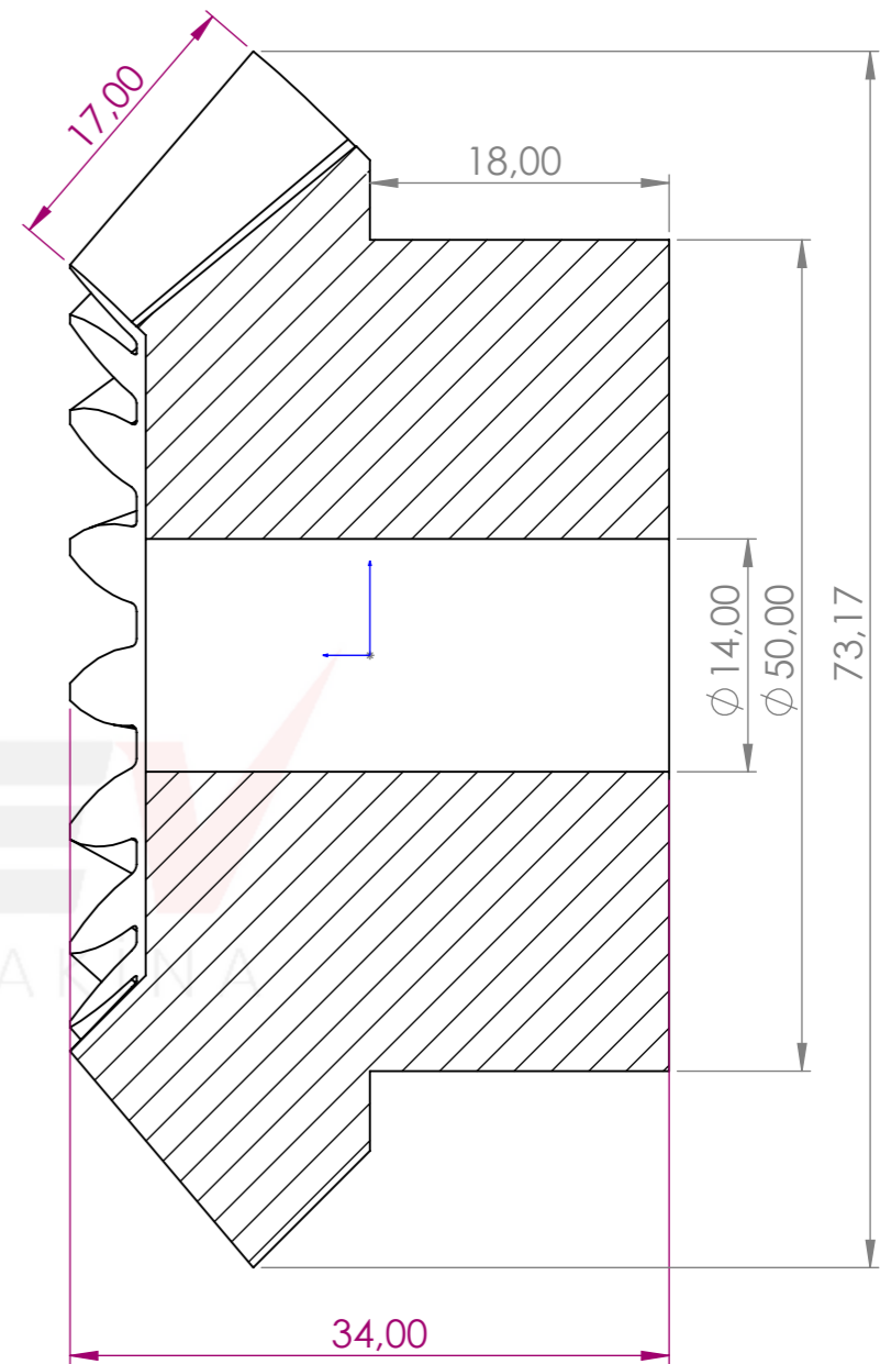
KESİT A-A ÖLÇEK 2 : 1
