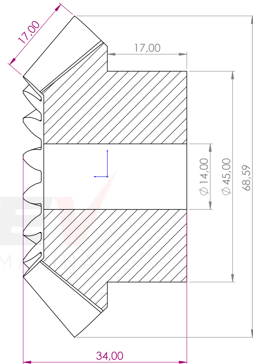
KESİT A-A ÖLÇEK 2 : 1
