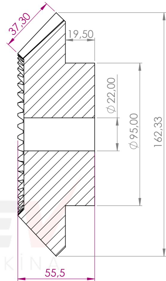
KESİT A-A ÖLÇEK 1 : 1.5
