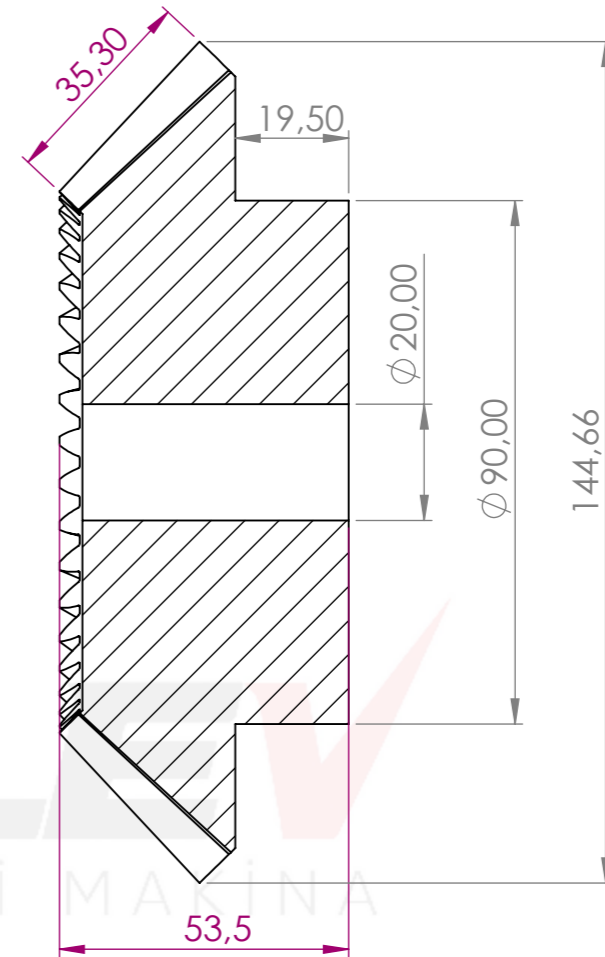
KESİT A-A ÖLÇEK 1 : 1.3
