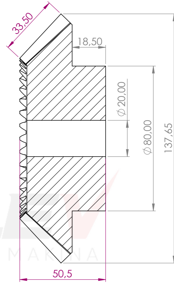
KESİT A-A ÖLÇEK 1 : 1.2
