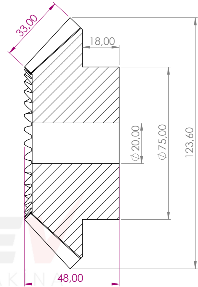
KESİT A-A ÖLÇEK 1 : 1.1
