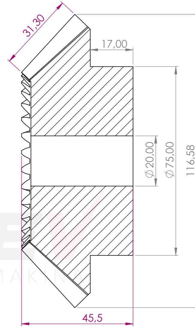
KESİT A-A ÖLÇEK 2 : 1.8
