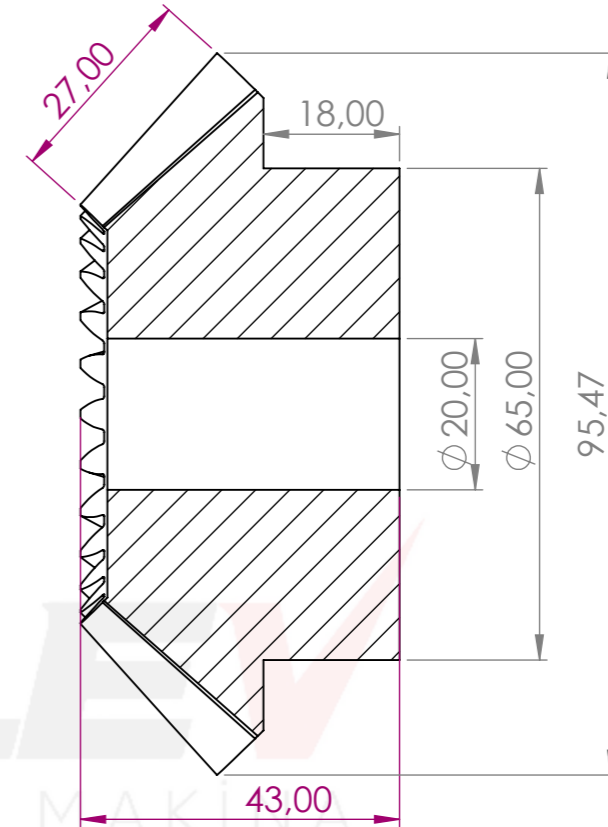
KESİT A-A
