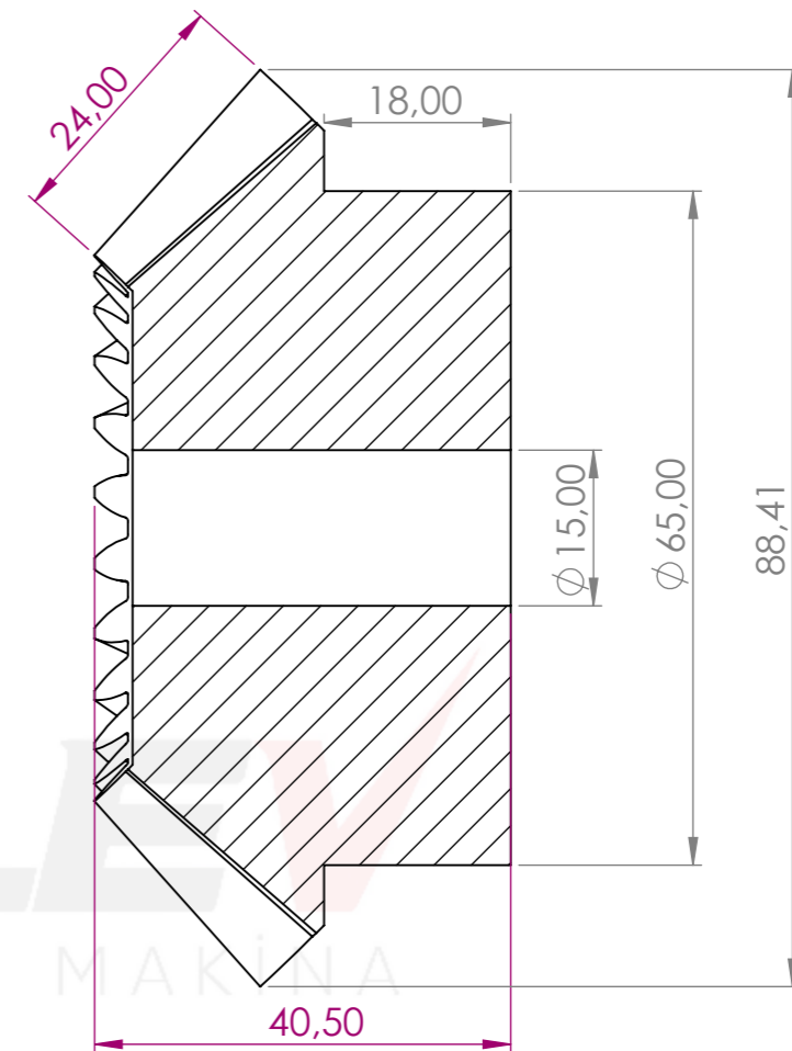
KESİT A-A ÖLÇEK 2 : 1.6
