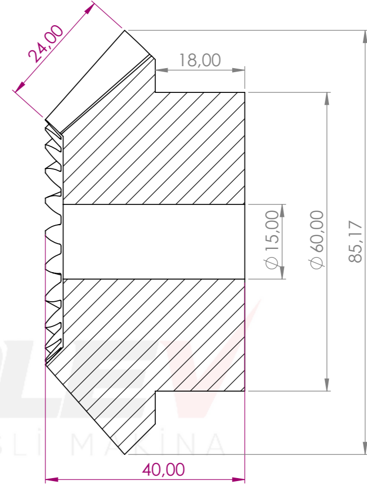
KESİT A-A ÖLÇEK 2 : 1.5
