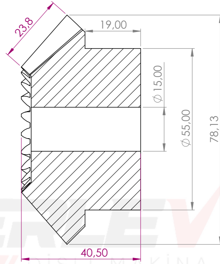
KESİT A-A ÖLÇEK 2 : 1.6
