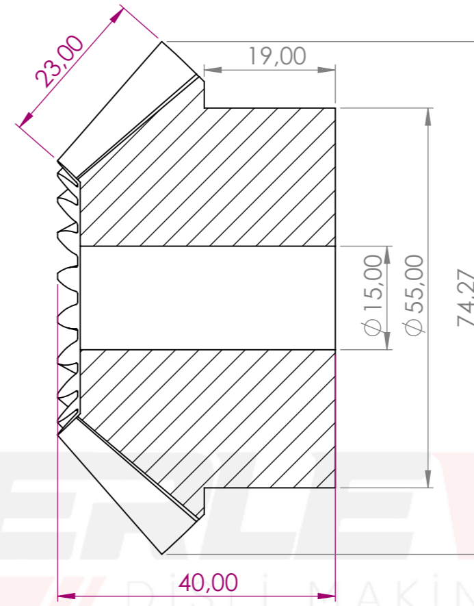
KESİT A-A ÖLÇEK 2 : 1.5
