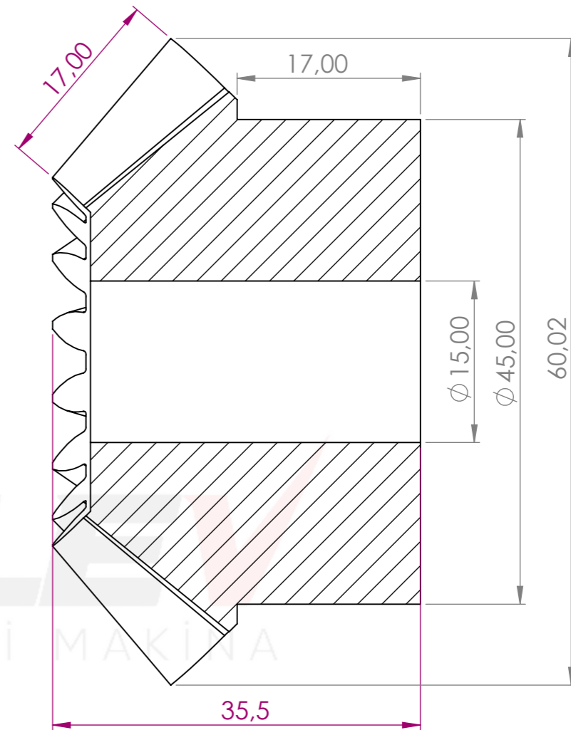
KESİT A-A ÖLÇEK 2 : 1
