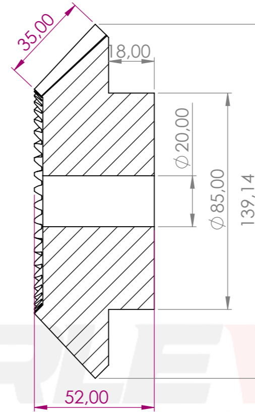
KESİT A-A ÖLÇEK 1 : 1.5
