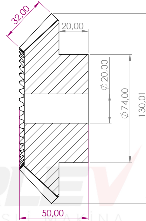
KESİT A-A ÖLÇEK 1 : 1.3
