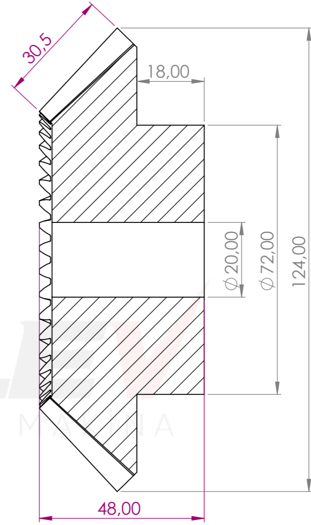
KESİT A-A ÖLÇEK 1:1
