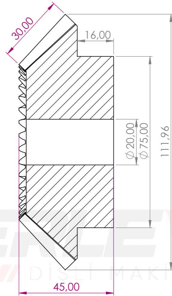
KESİT A-A
