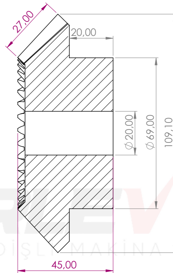
KESIT A-A
