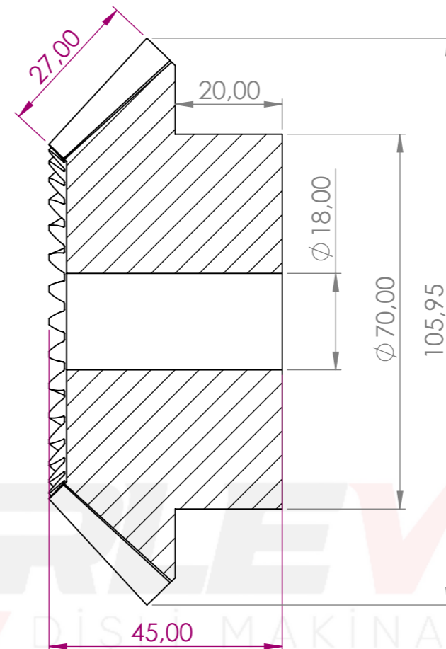
KESİT A-A
