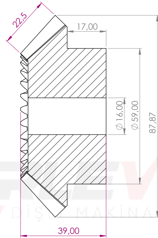
KESİT A-A ÖLÇEK 2 : 1.6
