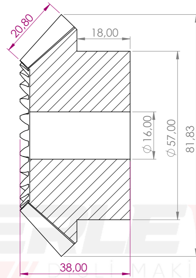
KESİT A-A ÖLÇEK 2 : 1.6
