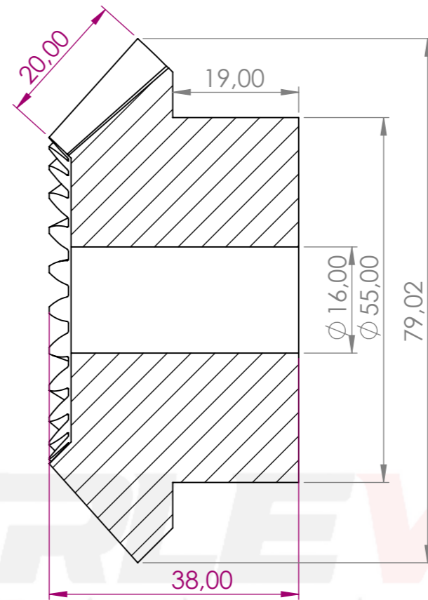
KESİT A-A ÖLÇEK 2 : 1.6
