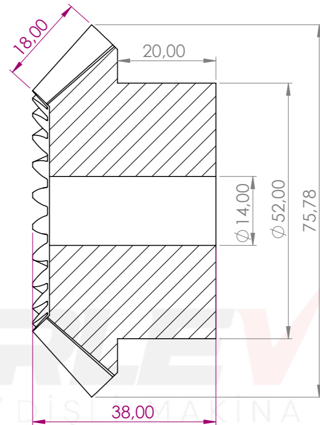
KESİT A-A ÖLÇEK 2 : 1.5
