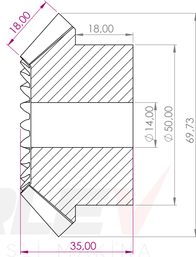
KESİT A-A ÖLÇEK 2 : 1.4
