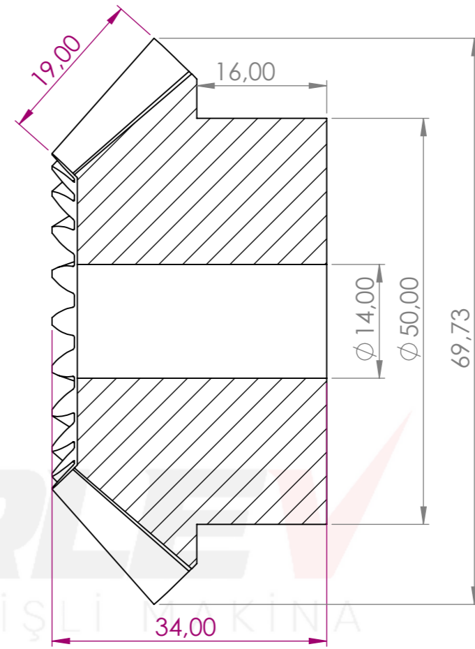
KESİT A-A ÖLÇEK 2 : 1.3
