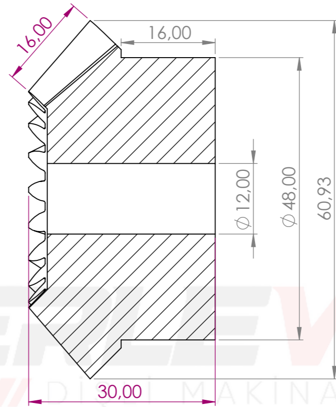
KESİT A-A ÖLÇEK 2 : 1.3
